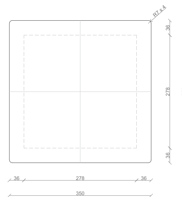
Pôdorýs
