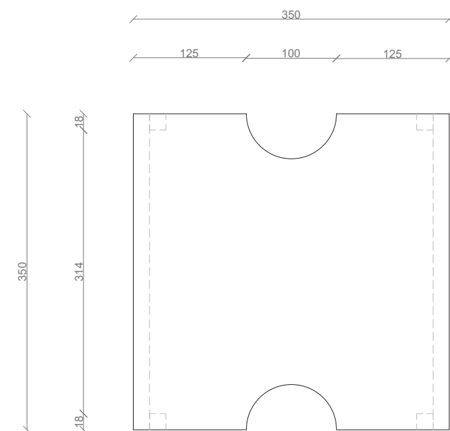
Nárys
