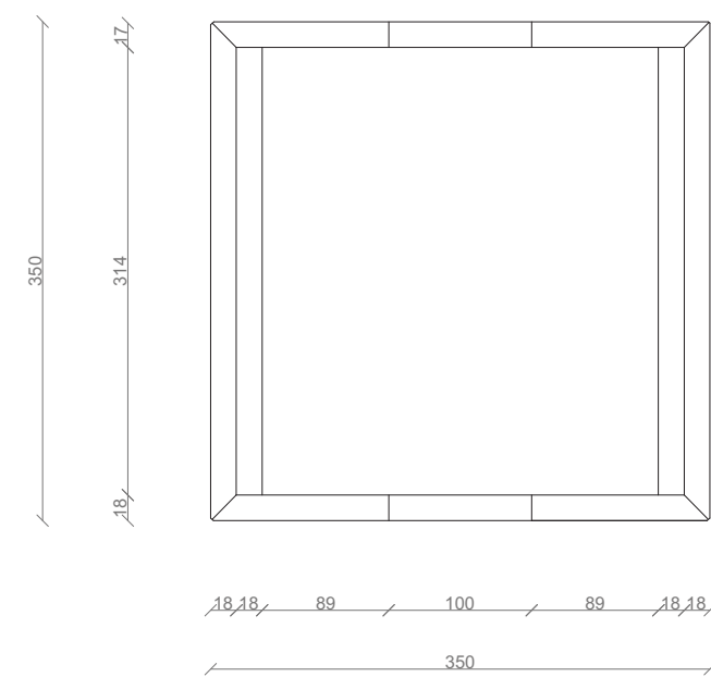
Pôdorýs
