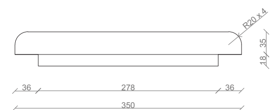
Nárys
